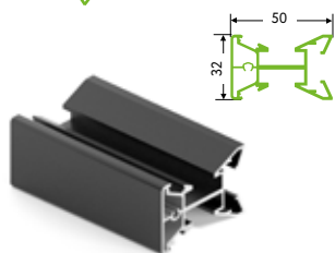
ST0851.VP540.BKSPC.CI STELLA Профиль вертикальный, L=5400 Длина - 5,4 м Цвет: черный матовый
