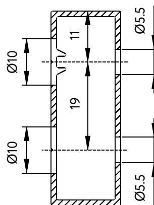
Сделайте отверстия в центре профиля для выкатных элементов
