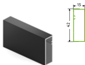
ST0884.VP540.BKSPC.CI STELLA Профиль для выкатных элементов, L=5400 Длина - 5,4 м Цвет: черный матовый
