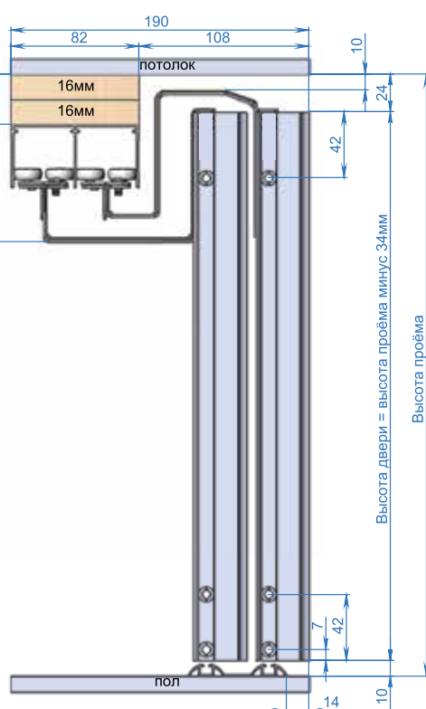
Скрытая установка направляющей верхней в проем
