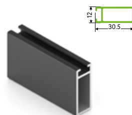
AA0717.VP540 Вешало алюминиевое Длина - 5,4 м Цвет: черный матовый
