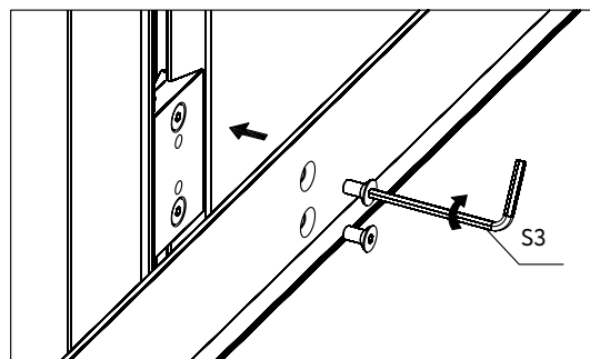
Закрепите полку со стеклом к закладной винтами
