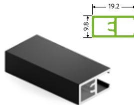
ST0853.VP540.BKSPC.CI STELLA Профиль для стеклянной полки, L=5400 Длина - 5,4 м Цвет: черный матовый
