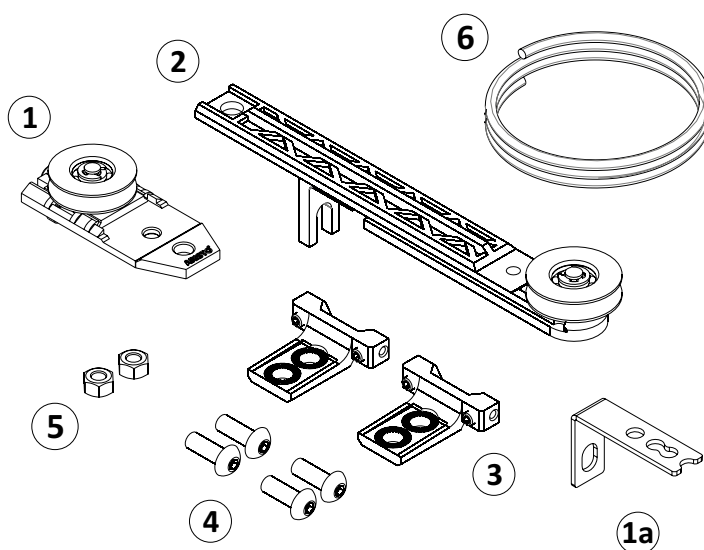
Ролик боковой для профиля Smart
