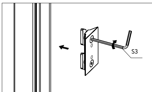
Зафиксируйте закладную в боковой части вертикального профиля, предварительно ослабив винты
