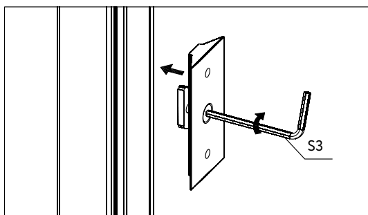
Зафиксируйте закладную в боковой части вертикального профиля, предварительно ослабив винты
