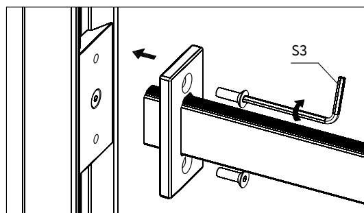
Закрепите штангу с креплением к закладной винтами
