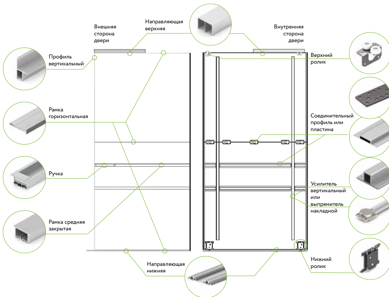
Скрытая установка направляющей верхней
