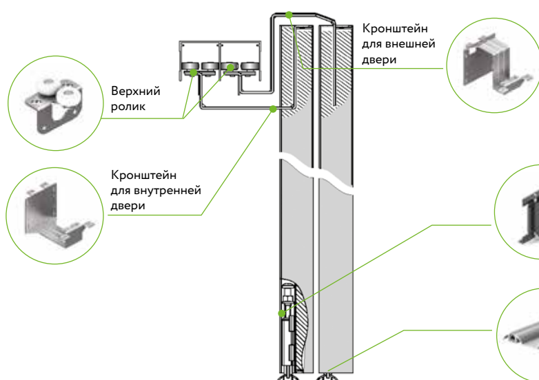
Скрытая установка направляющей верхней
